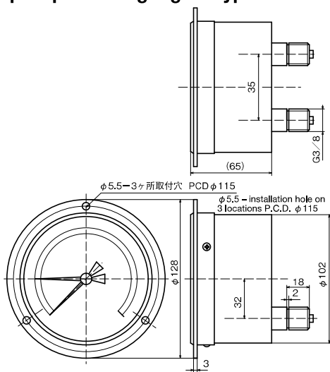
複針ゲージ D型 FA13-4 Duplex pressure gauge D type FA13-4
