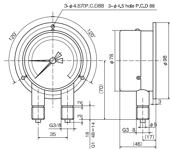
複針ゲージ B型 FA12-3 Duplex pressure gauge B type FA12-3
