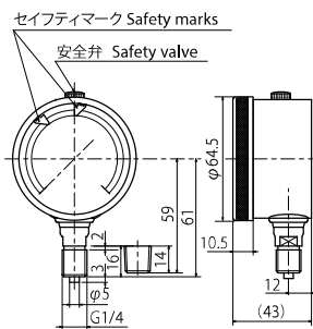
SG11 A型ゲージ 図面 SG11 A type Gauge: Drawings
