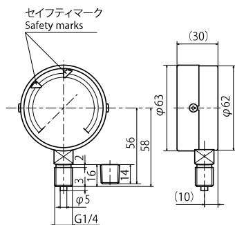
SP11 A型ゲージ 図面 SP11 A type Gauge: Drawings
