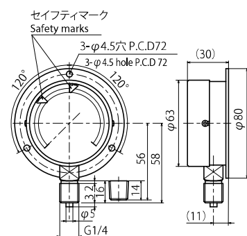
SP12 B型ゲージ 図面 SP12 B type Gauge: Drawings
