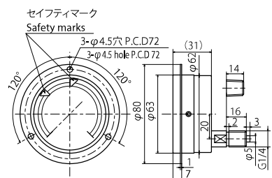
SP13 D型ゲージ 図面 SP13 D type Gauge: Drawings
